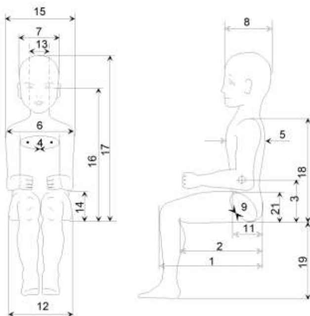
Rysunek 1 Podstawowe wymiary manekina – dodatek 1 do załącznika 8, Regulaminu EKG ONZ nr 44
